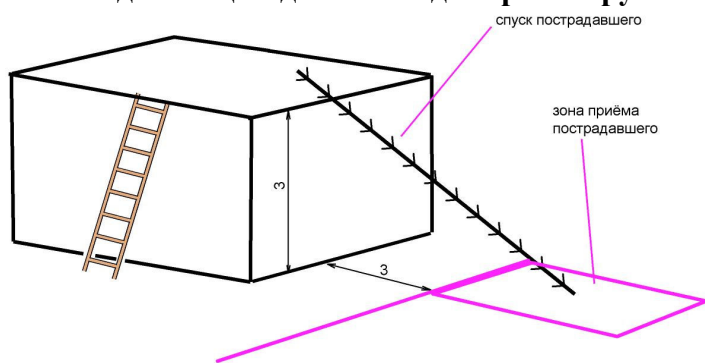
Схема дистанции для команд старшей группы
