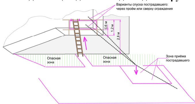
Схема дистанции для команд младшей группы
